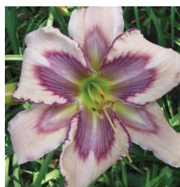
POLAR VORTEX (Howard-R., 2014)
